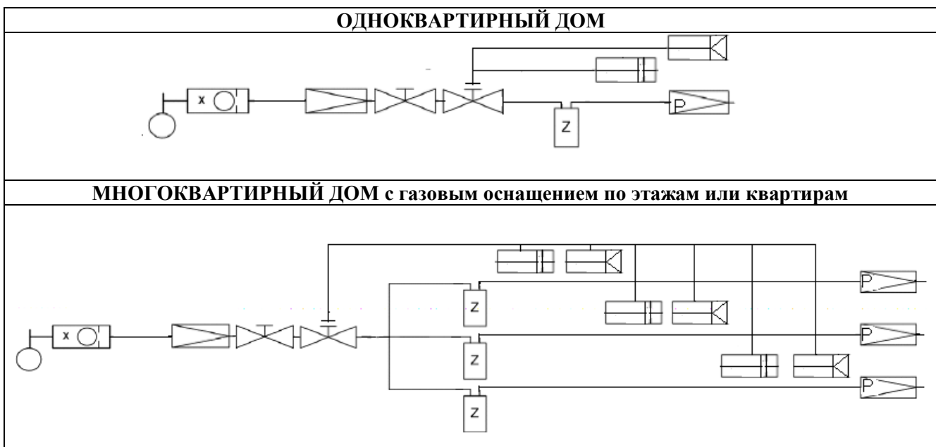
Рис. Е.2. Активные меры безопасности при давлении в наружном газопроводе \geq 0,005 МПа до 0,6 МПа и приборы, регулирующие давление газа.
