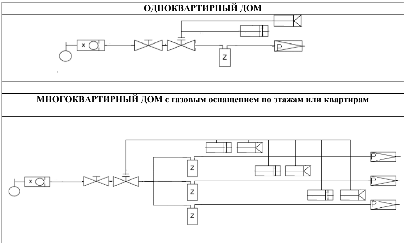
Рис. Е.1. Активные меры безопасности при давлении в наружном газопроводе >0,0015 МПа (150 мм вод.ст.) до 0,005 МПа и приборы, регулирующие давление газа.
